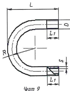
ОТВОД 180° КАЛАНЧ РЕЗЬБОВОЙ
