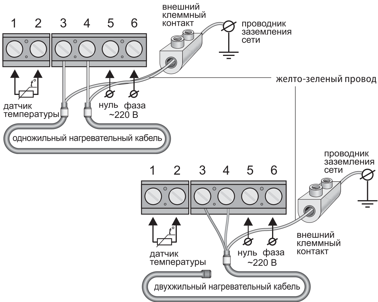
Рис. 4. Схема подключения терморегулятора TR 140 к трехпроводной электрической сети
